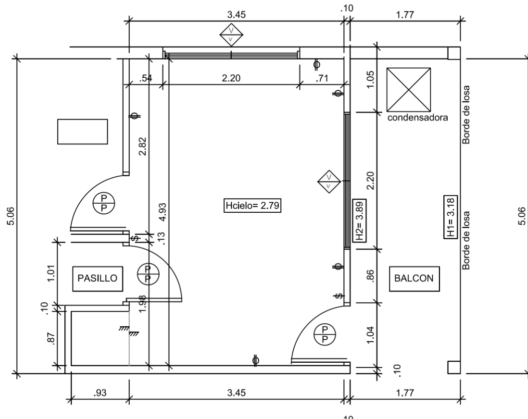
PLANTA EXISTENTE AREA 1
