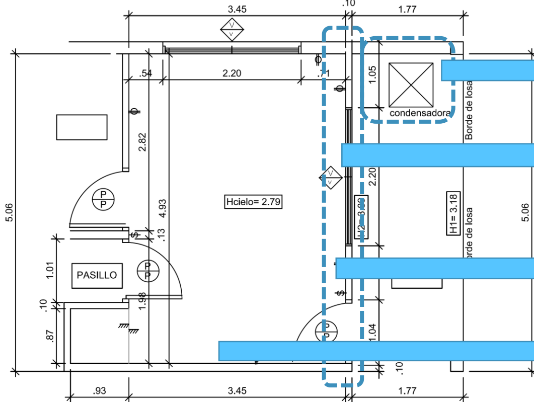
PLANTA EXISTENTE AREA 1
